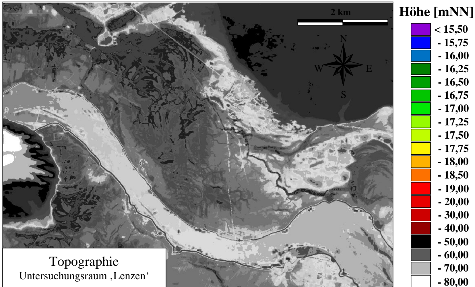
Abb. 5: Topographie des Untersuchungsraumes (Ausschnitt)
