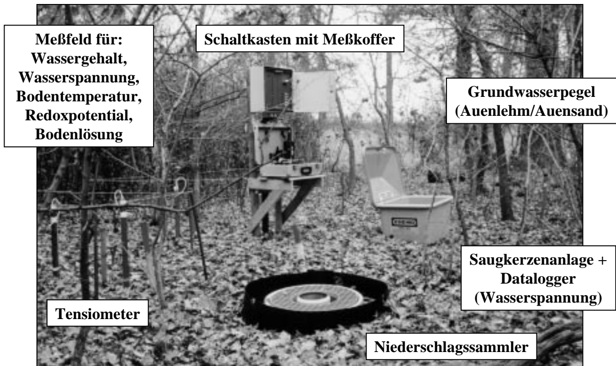
Foto 10: Darstellung der Meßapparatur am Teststandort ,EW'
